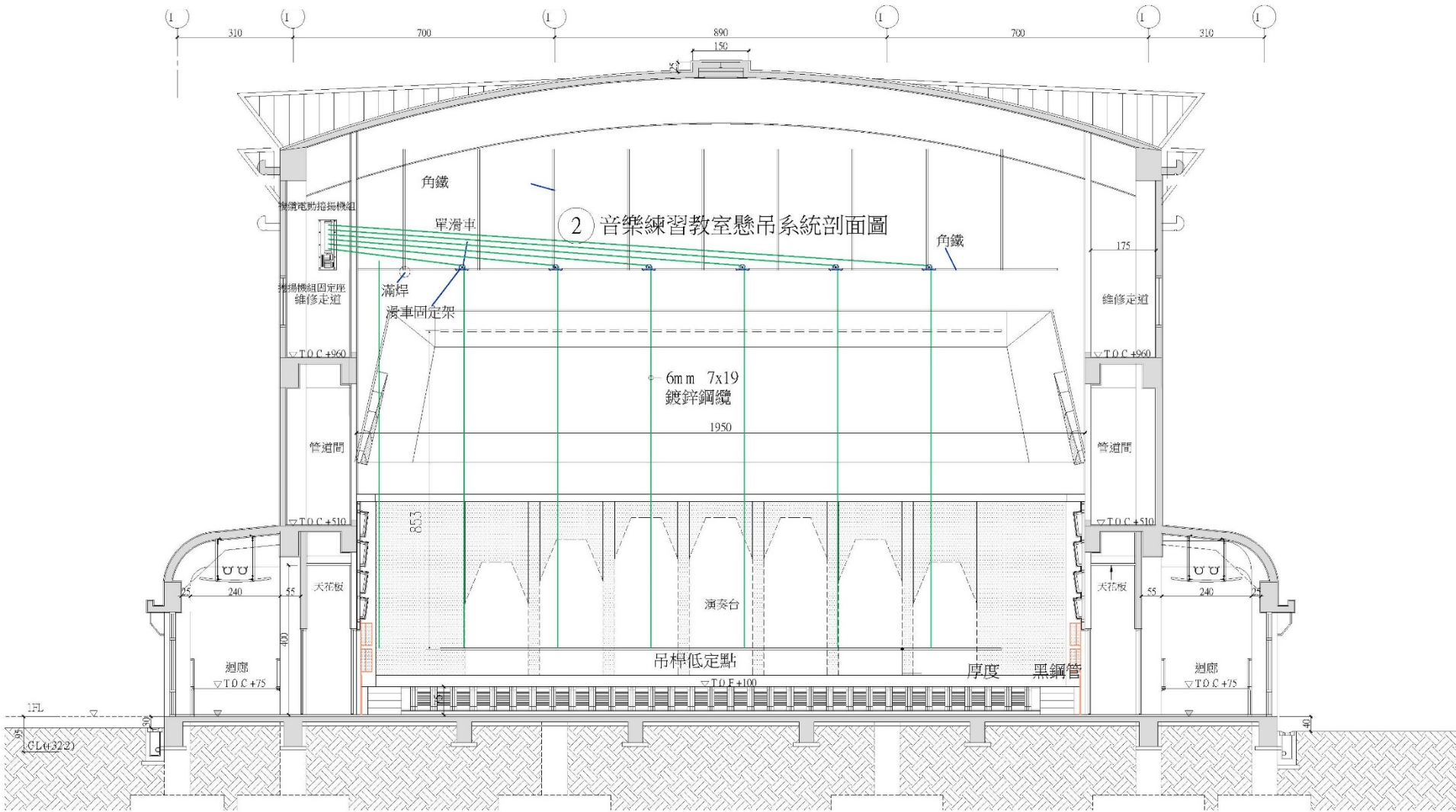
懸吊系統剖面圖
